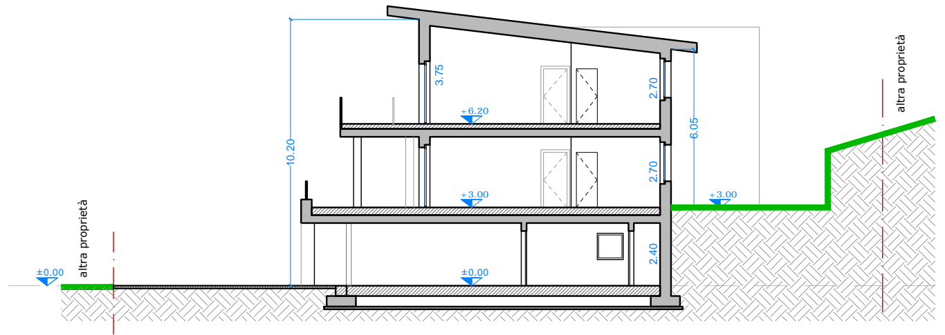
sezione A-A
